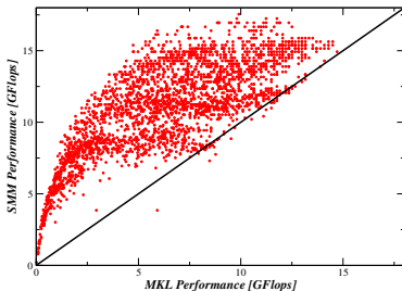
Σχήμα: Σύγκριση απόδοσης libSMM vs MKL για 1 \leq N/M/K \leq 24 .
